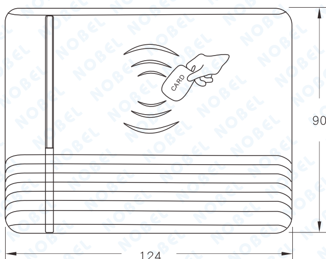
正視圖
