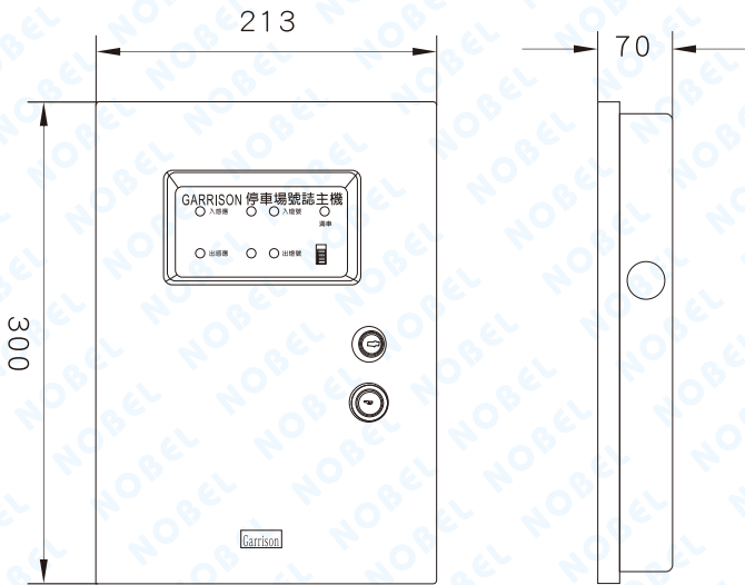
正視圖
