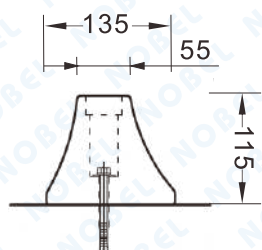
側立面圖
