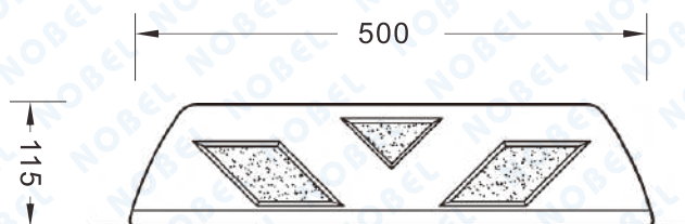
正視圖
