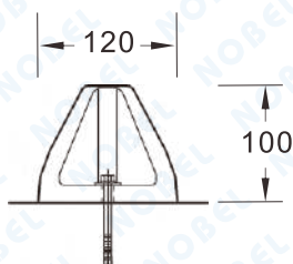
側立面圖
