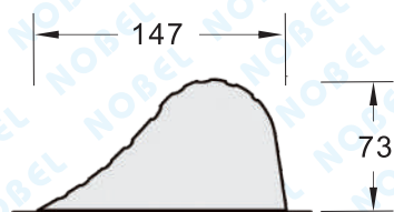
側立面圖
