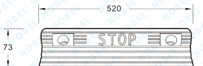
正視圖
