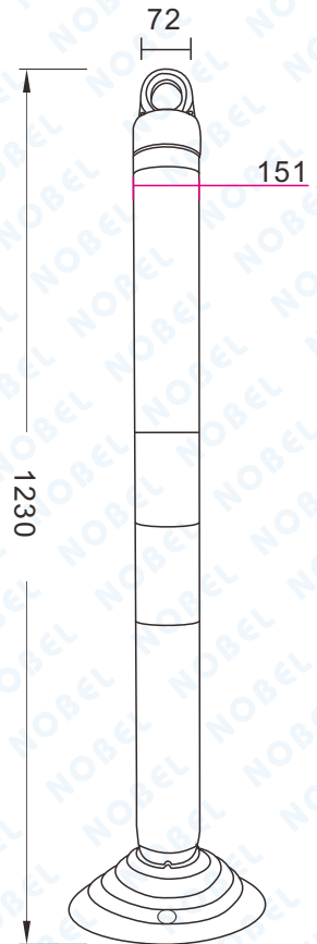
側立面圖
