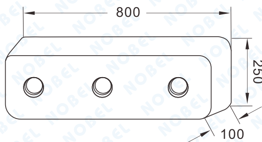
E-80 卸貨塊 正視圖
