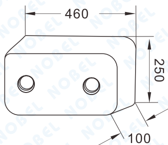
E-45 卸貨塊 正視圖
